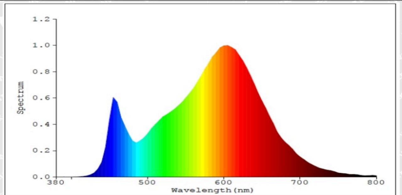
Model: 97260 (3000K)
