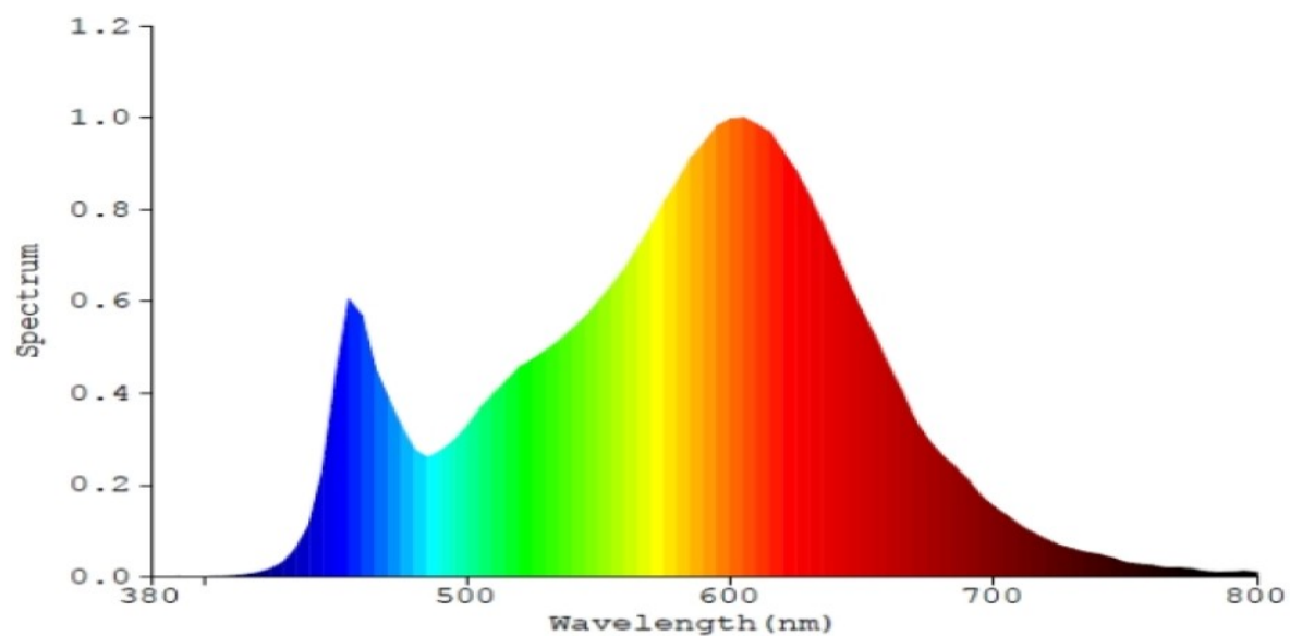
Model: 97240 (3000K)
