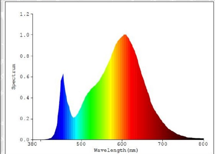
Model: 97200 (3000K)
